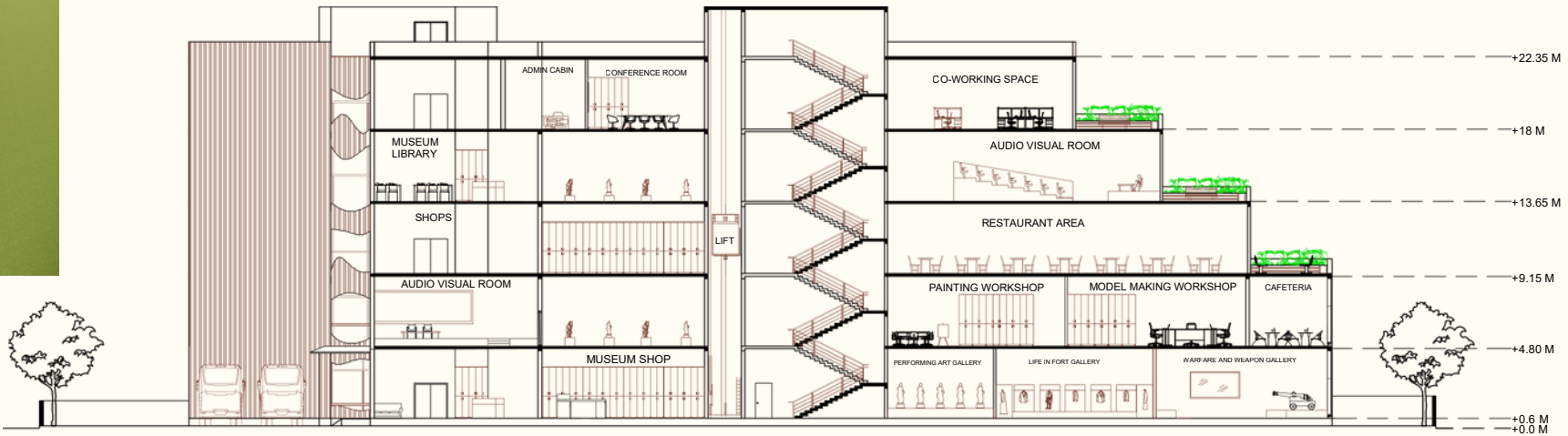
SECTION A-A'
